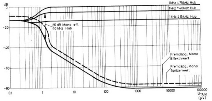
Fremdspannungsverlauf FM in Abhängigkeit von der Antennenspannung
